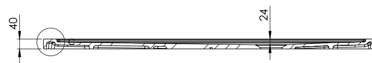
SECTION A-A
